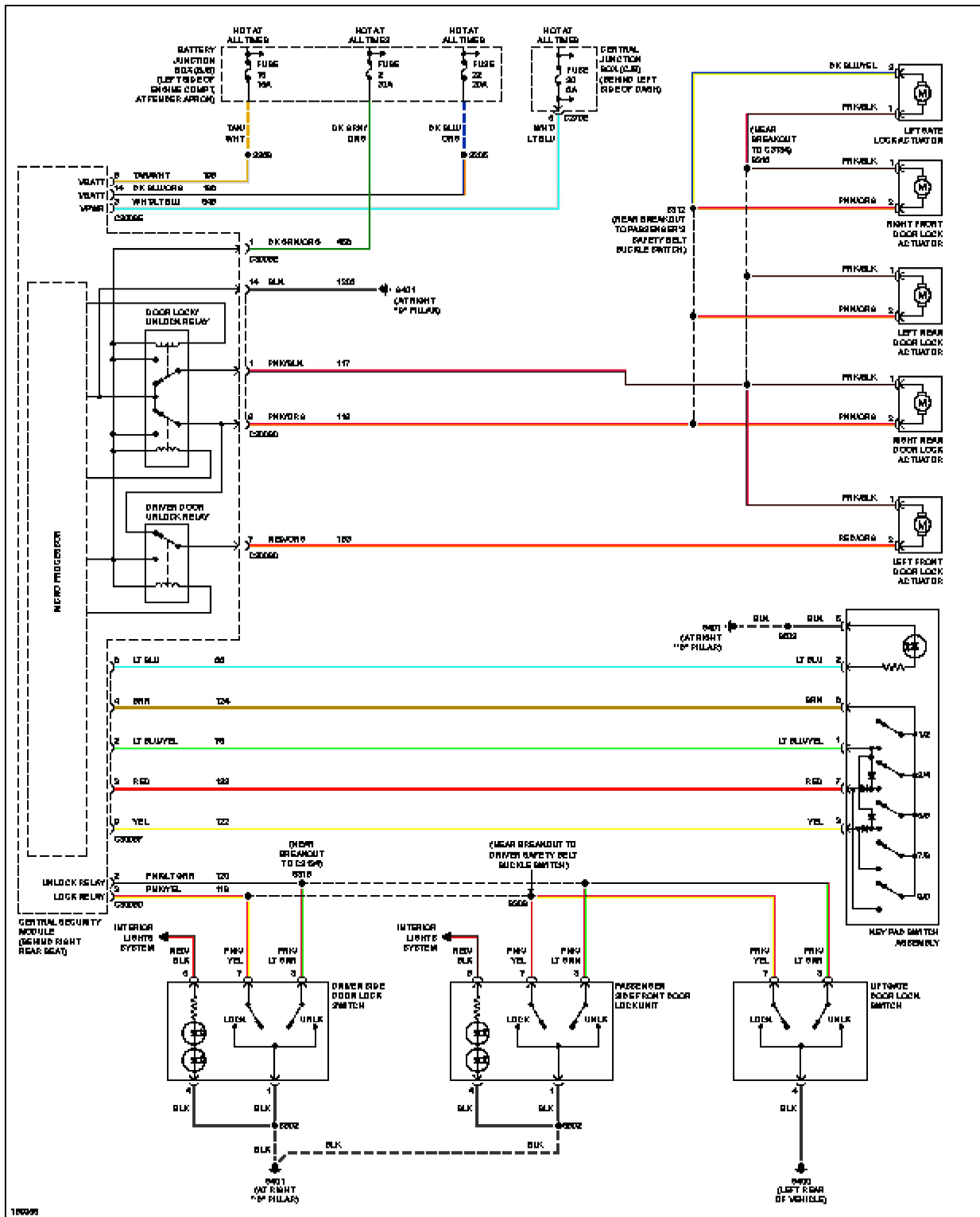
Fig. 47: Power Door Locks Circuit
