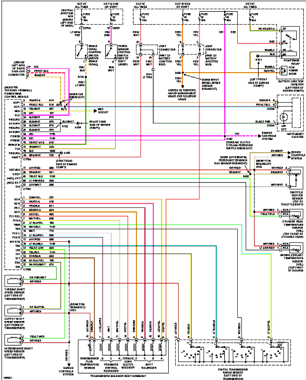
Fig. 67: A/T Circuit
