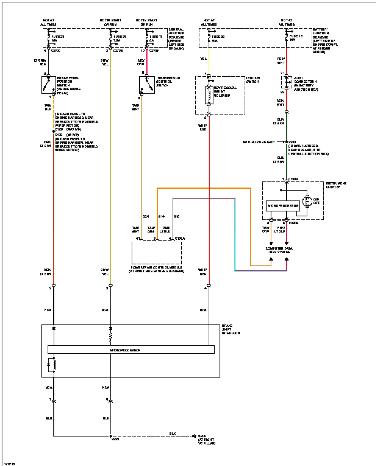
Fig. 60: Shift Interlock Circuit
